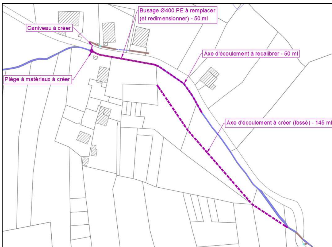
Proposition de travaux – Dysfonctionnement n°1 – Chez les Bauds
