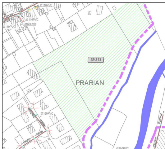
Extrait du plan « Diagnostic hydraulique » du SGEP
