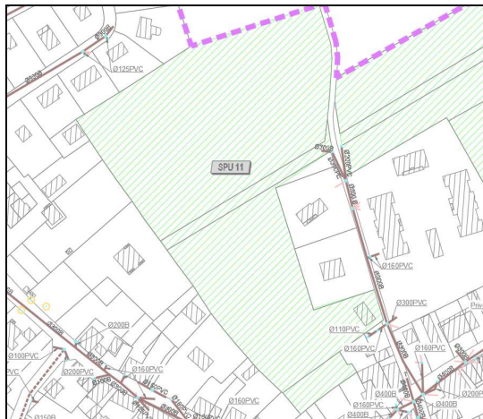
Extrait du plan « Diagnostic hydraulique » du SGEF
