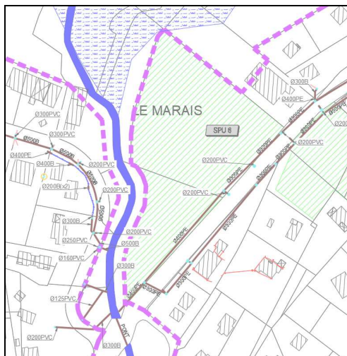
Extrait du plan « Diagnostic hydraulique » du SGEP
