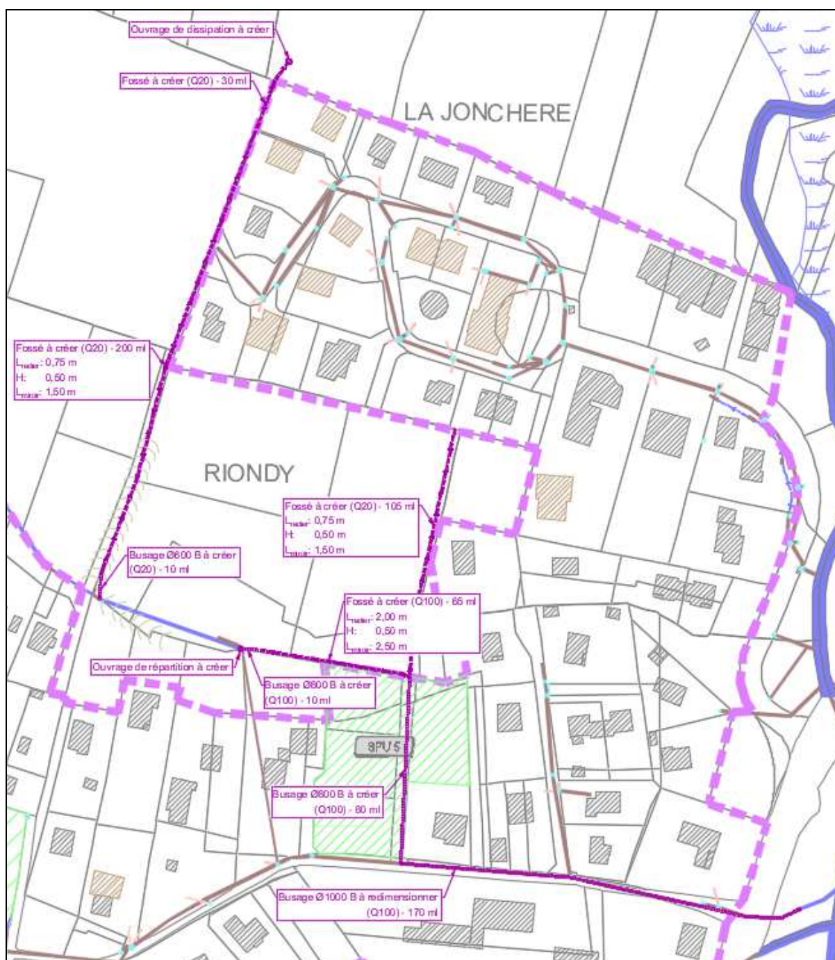
Proposition de travaux – Dysfonctionnement n°3 – Riondy, La Jonchère
