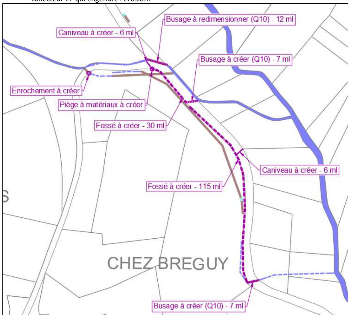
Proposition de travaux – Dysfonctionnement n°2 – Chemin de Chez Ranquin
