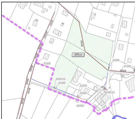
Extrait du plan « Diagnostic hydraulique » du SGEP
