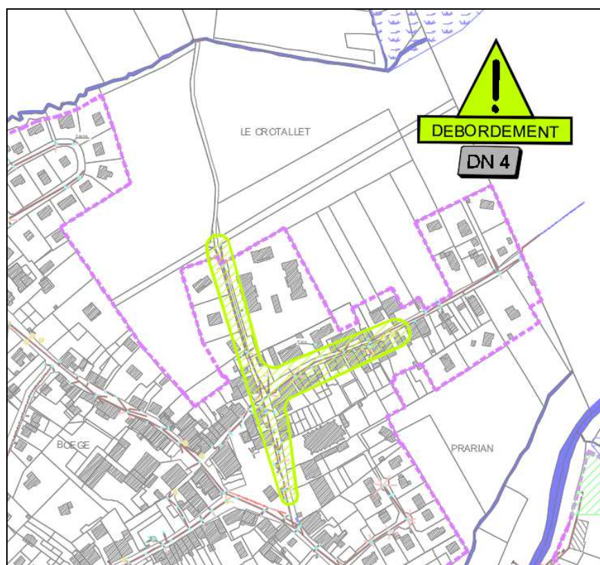
Extrait du plan « Diagnostic hydraulique » du SGEP
