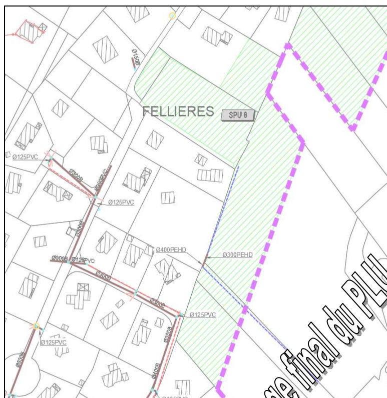
Extrait du plan « Diagnostic hydraulique » du SPU 8
