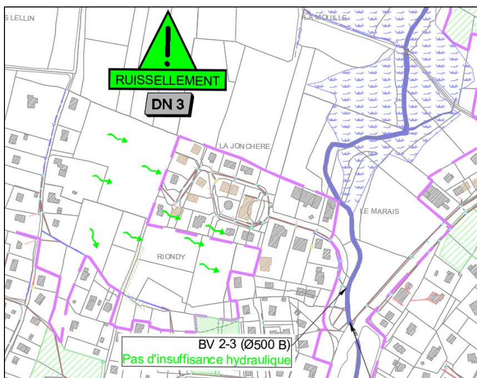
Extrait du plan « Diagnostic hydraulique » du SGEP
